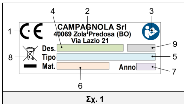
Ακολουθεί φάξ Ομοίωση της πινακίδας CE (*)
